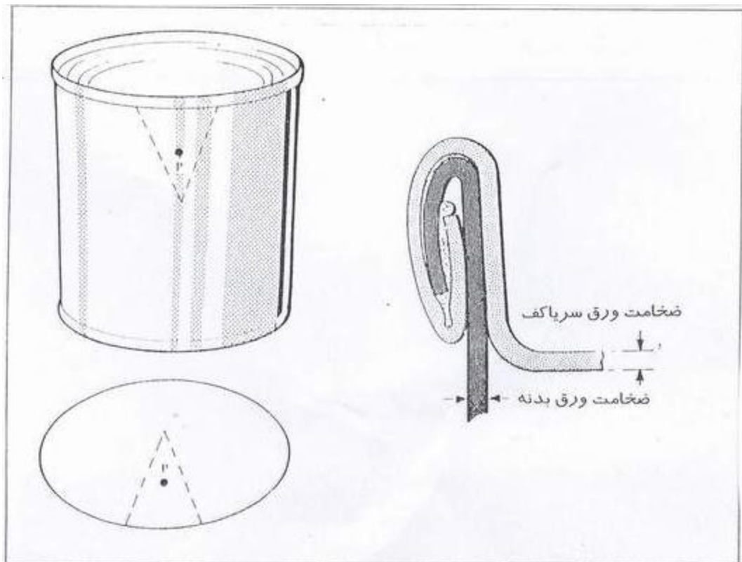
شکل ۱۸- محل اندازه گیری ضخامت بدنه و سرباکف
